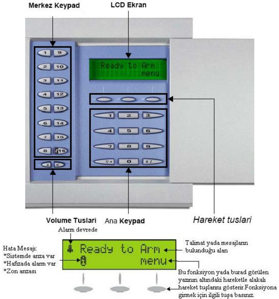
Şekil 3.16: Display
