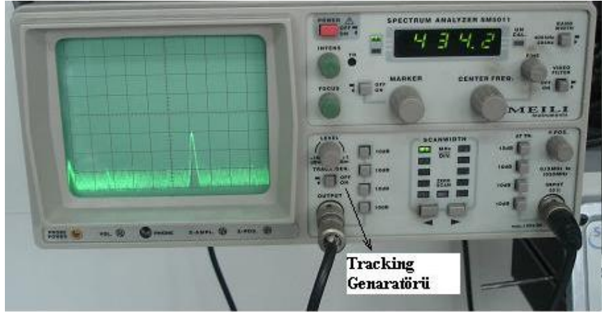
Şekil 1.10a: Hibrit alıcının spektrum analizöre bağlanması
