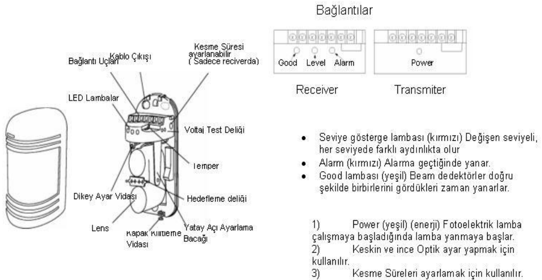
Şekil 3.45: Beam dedektörü
