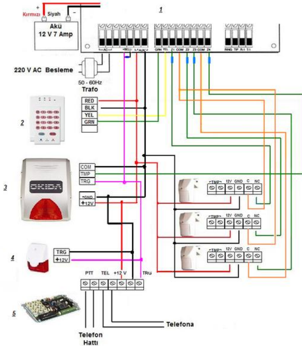
Şekil 3.47: Kontrol paneli bağlantısı
