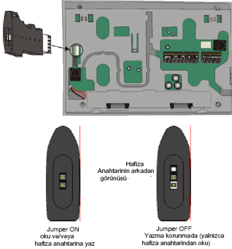
Şekil 2.1: Hafıza anahtarından konsola konsoldan hafızaya program yükleme
