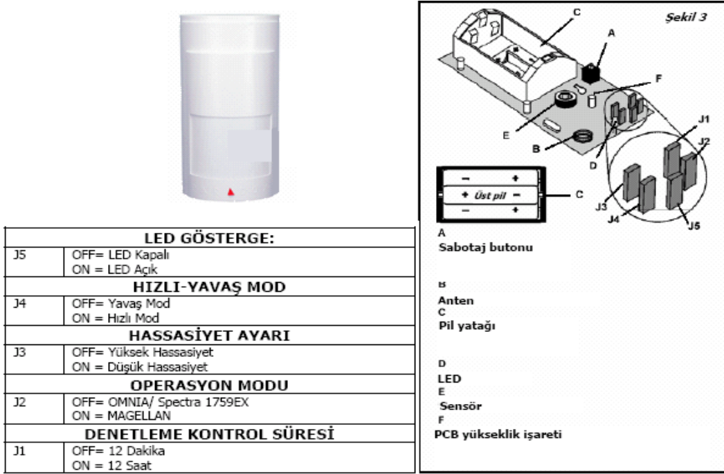
Şekil 3.29: Dual elementli hareket dedektörü ve iç yapısı
