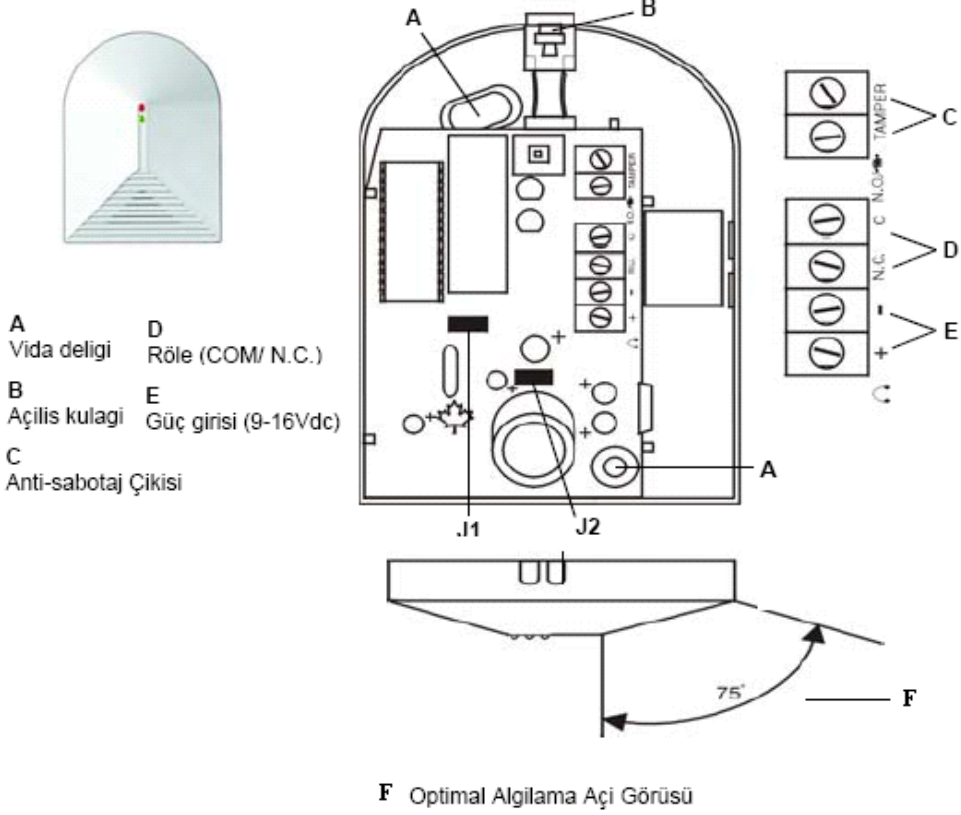
Şekil 3.36: Cam kırılma dedektörü
