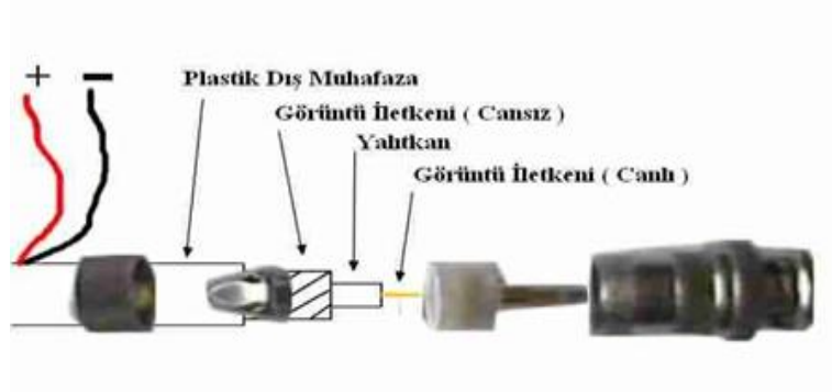
Resim 3.18: Koaksiyel kablonun BNC'ye montajı
