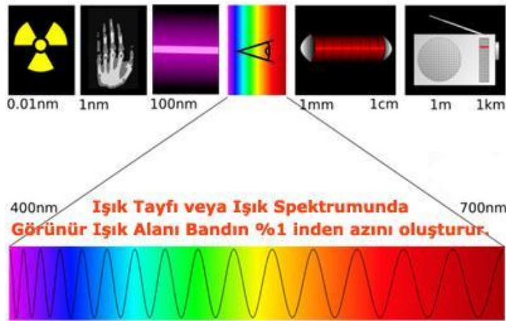
Resim3.1: Işık spektrumu
