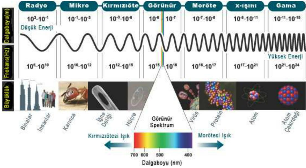
Resim3.7: Elektromanyetik spektrum
