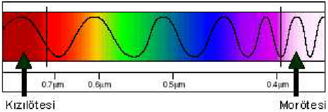
Şekil 3.1:Görünürışık spektrumu
