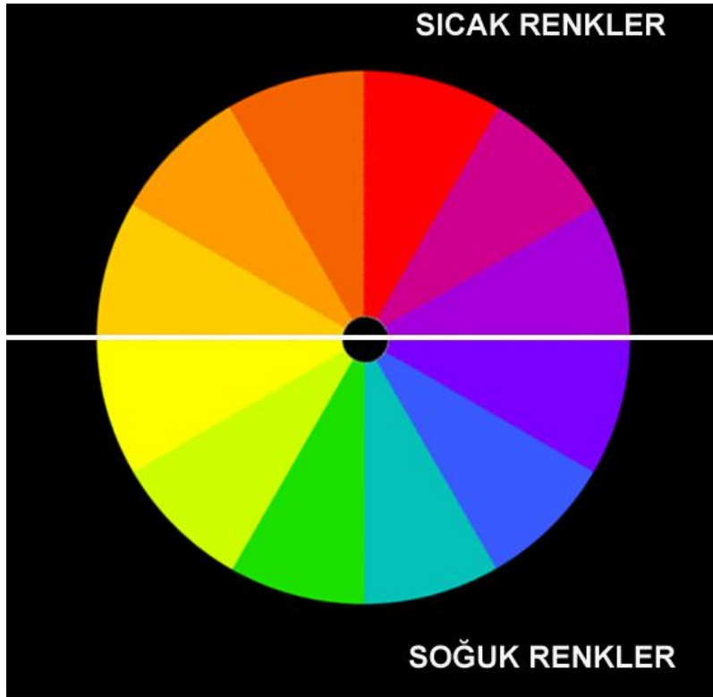
Şekil 3.3 : Renk tablosu
