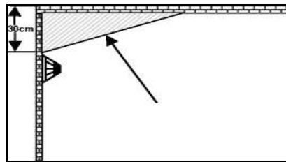
Şekil 2.30: Ölü bölge
