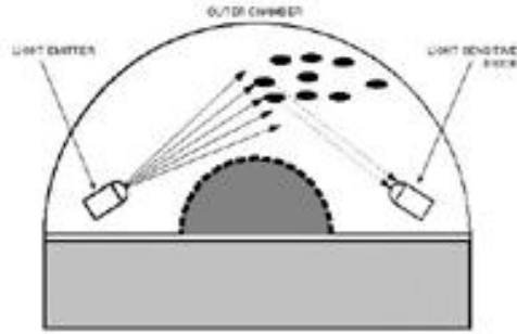
Şekil 2.8: Optik duman detektörü prensip şeması
