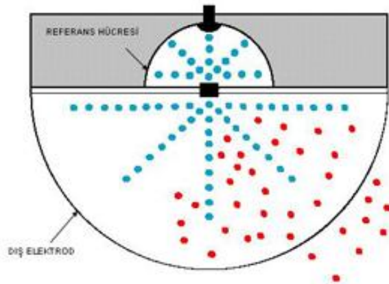
Şekil 2.7: İyonizasyon duman detektörü prensip şeması
