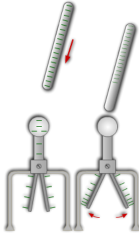
Şekil 45: Yüğü elektroskop yükünden büyük olan bir cismin elektroskop yapraklarına etkisi
