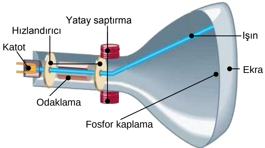
Şekil 41: Katot ışınlı tüp modeli
