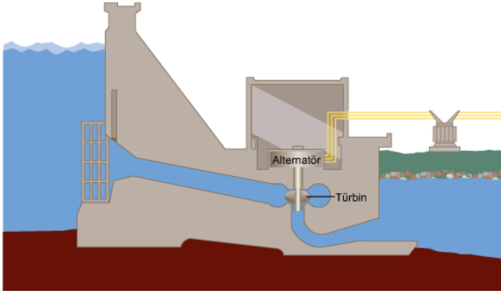
Şekil 5: Hidrolik santral modeli
