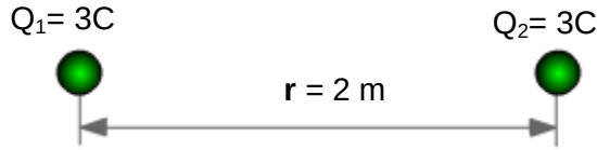
Şekil 21: Pozitif yükler
