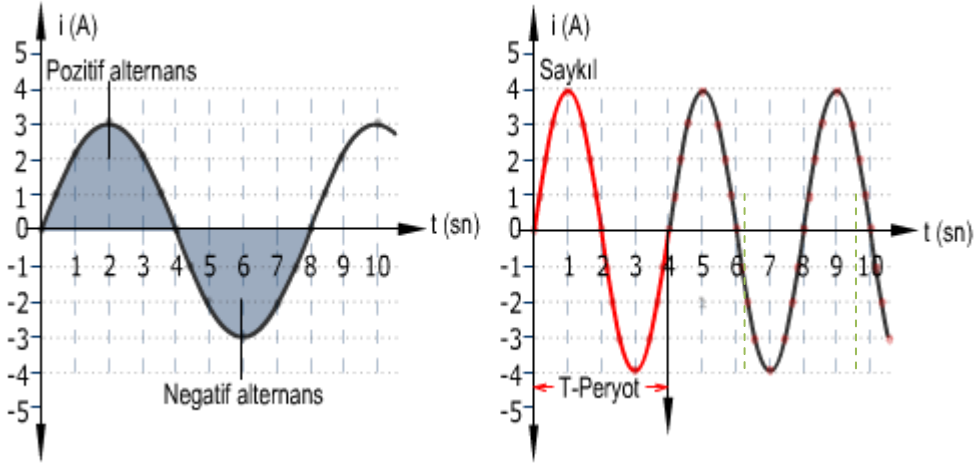
Şekil 62: Alternatif akım eğrileri
